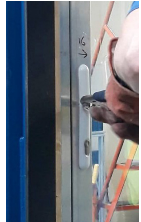
PAS 24 test
